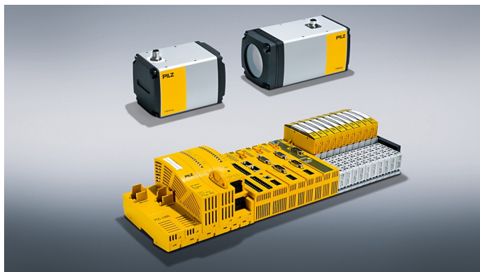
Bildtext: Den nya kantpressmodulen från Pilz förenklar programmeringen av den dynamiska muting-processen avsevärt för det kamerabaserade skyddssystemet PSEnvip 2. (Foto: © Pilz GmbH & Co. KG)
