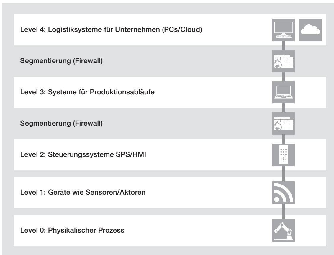
Abbildung 13: Netzwerksegmentierung anhand des Purdue-Modells
